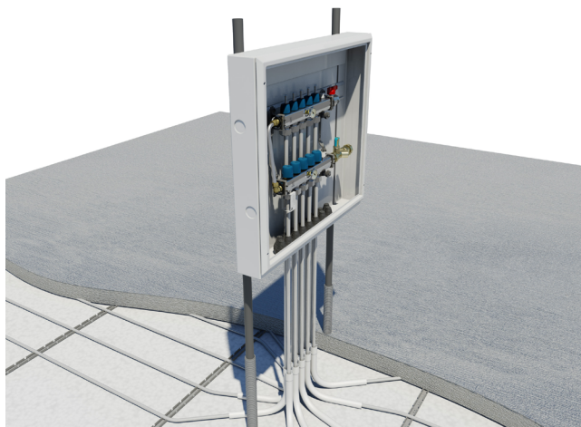
LK Kaappiteline L2 ja LK Jakotukkikaappi
